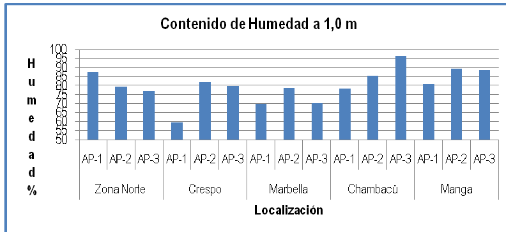
Gráfica 3. Contenido de Humedad muestras recuperadas a 1.0 m de profundidad
