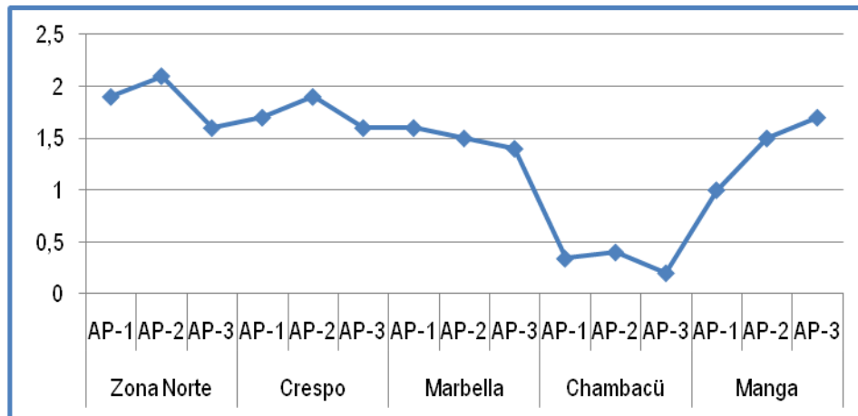
Gráfica 10. Determinación de Salinidad a muestras recuperadas a 0.5 m de profundidad
