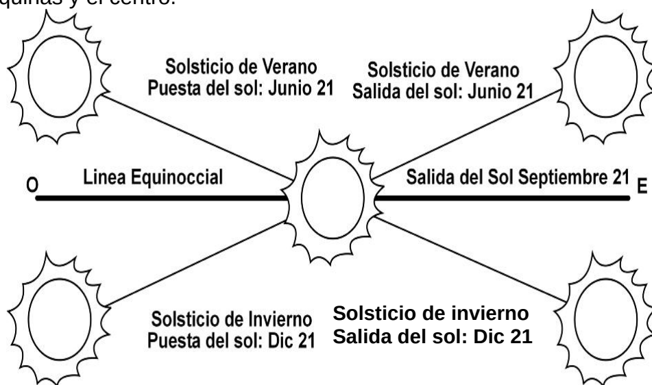
Figura 1. Las cuatro “esquinas del cielo” en los solsticios y el punto central al pasar el sol por el cenit, basado en Villa Rojas.
