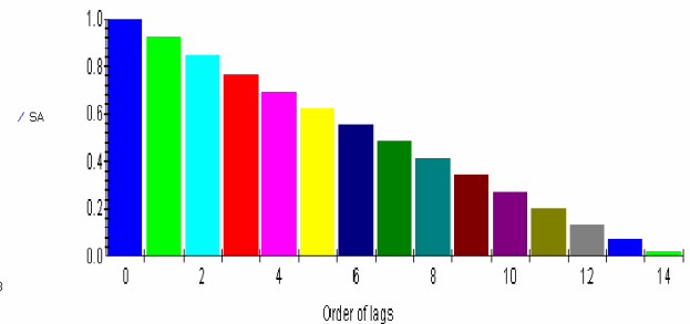
Función de Autocorrelación de PIBR
