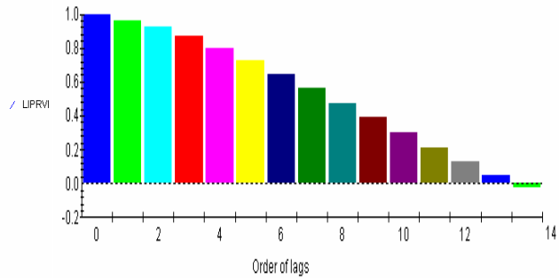
Función de Autocorrelación de LIPRVI
