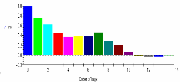
Función de Autocorrelación de INF
