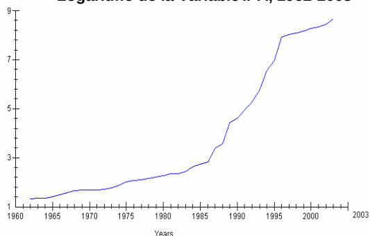
Logaritmo de la Variable IPRA, 1962-2003
