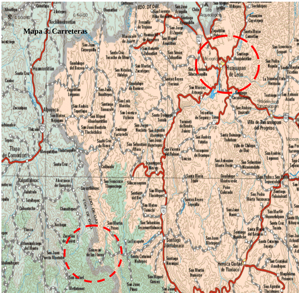
Mapa de carreteras pavimentadas y de terracería de la Región de la Mixteca
