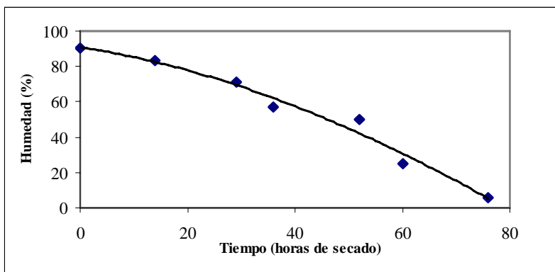
Figura 2: Curva de secado de orégano en el secador solar "Agrosol" de 20 m 2
