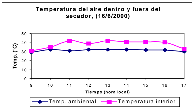
Figura 1: Temperaturas del aire dentro y fuera del secador
