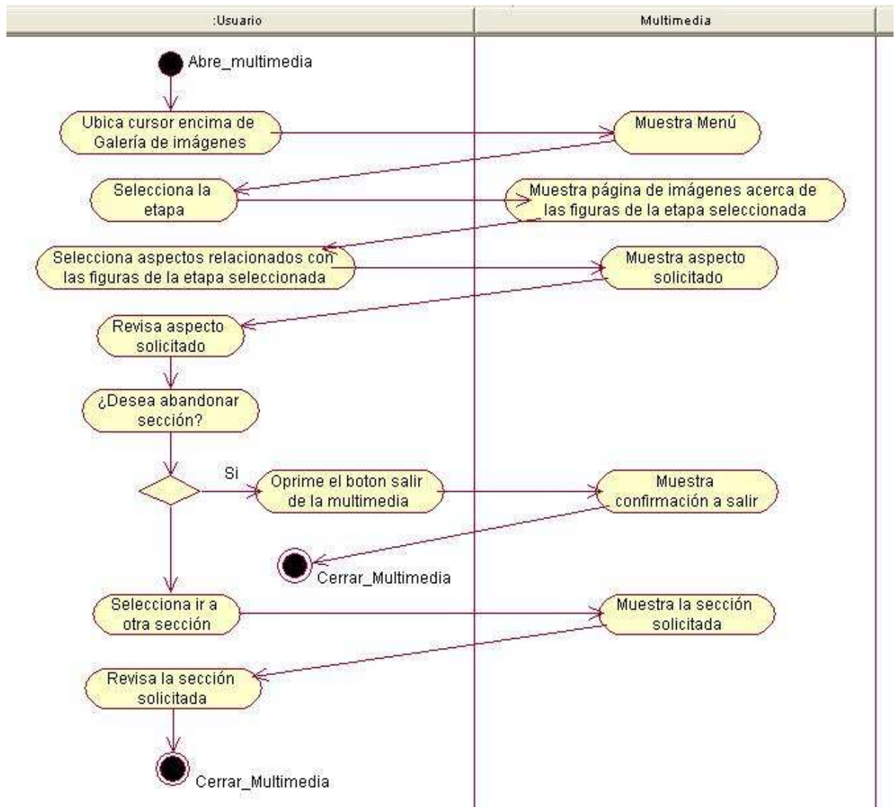
Diagrama de actividades del caso de uso revisar galería de imágenes y biografías.
